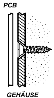
Abbildung B.4: Schraubenposition bei Montage
