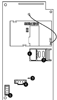
Abbildung 1.6: Mobiltelefon Kommunikationsmodul
