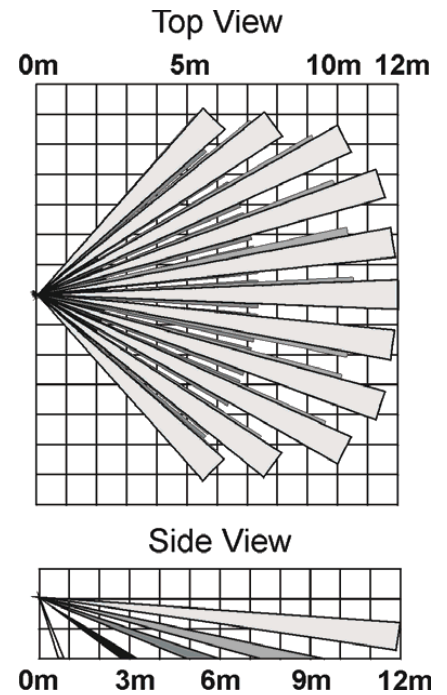
Figura B.2: Diagrammi copertura lenti MS845
