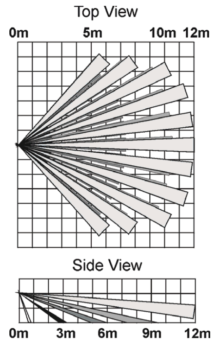
Figure B.2: Abbildung B.2: Linsenbedeckungsdiagramme MS845
