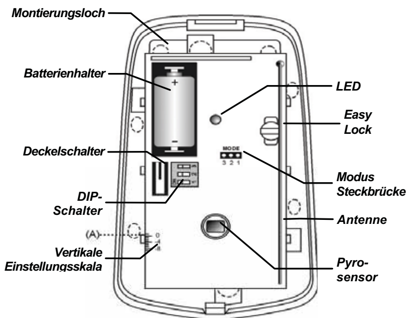
Abbildung B.1: PIR Sensor ohne Abdeckung MS845
