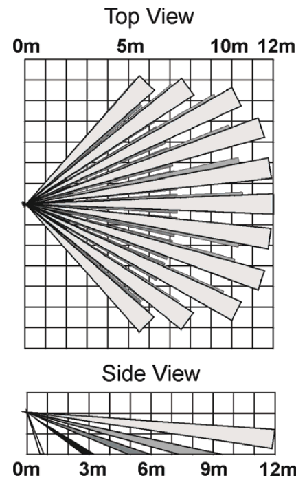
Figura B.2: Diagramas de Cobertura MS845
