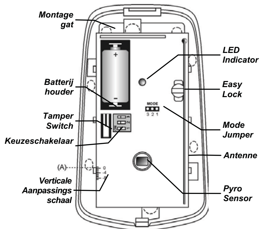
Figuur B.1: PIR Sensor zonder cover
