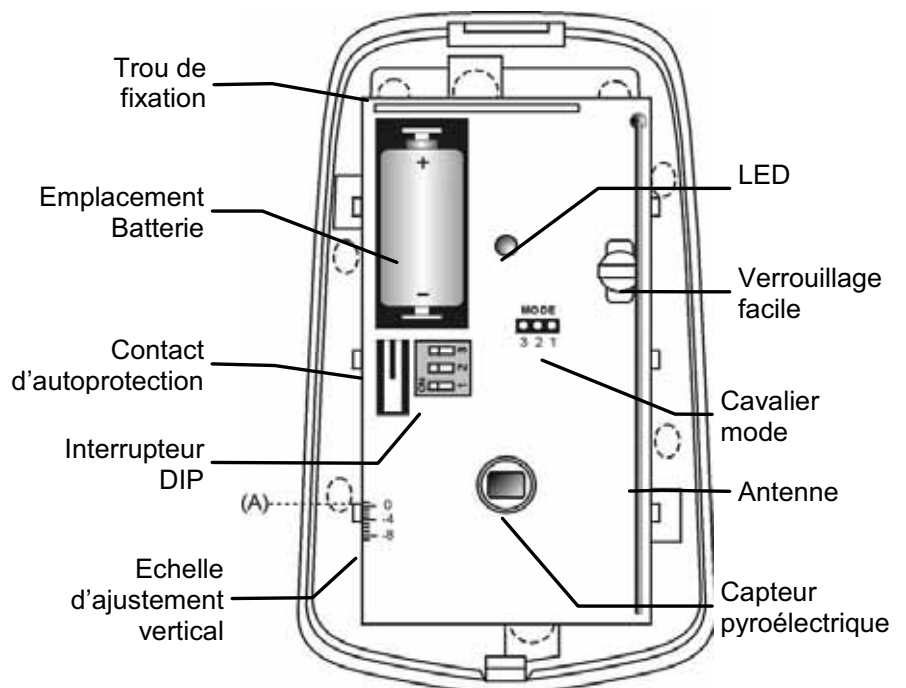
Figure B.1: Détecteurs IRP sans couvercles MS845
