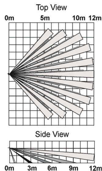
Figuur B.2: Dekking van de Lens Diagrammen
