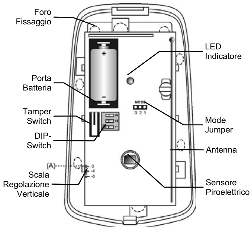
Figura B.1: Sensore PIR senza copertura MS845
